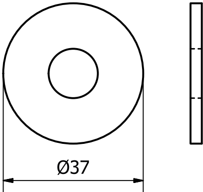
DIN 9021 - 13
