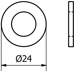
DIN 125 A - 13
