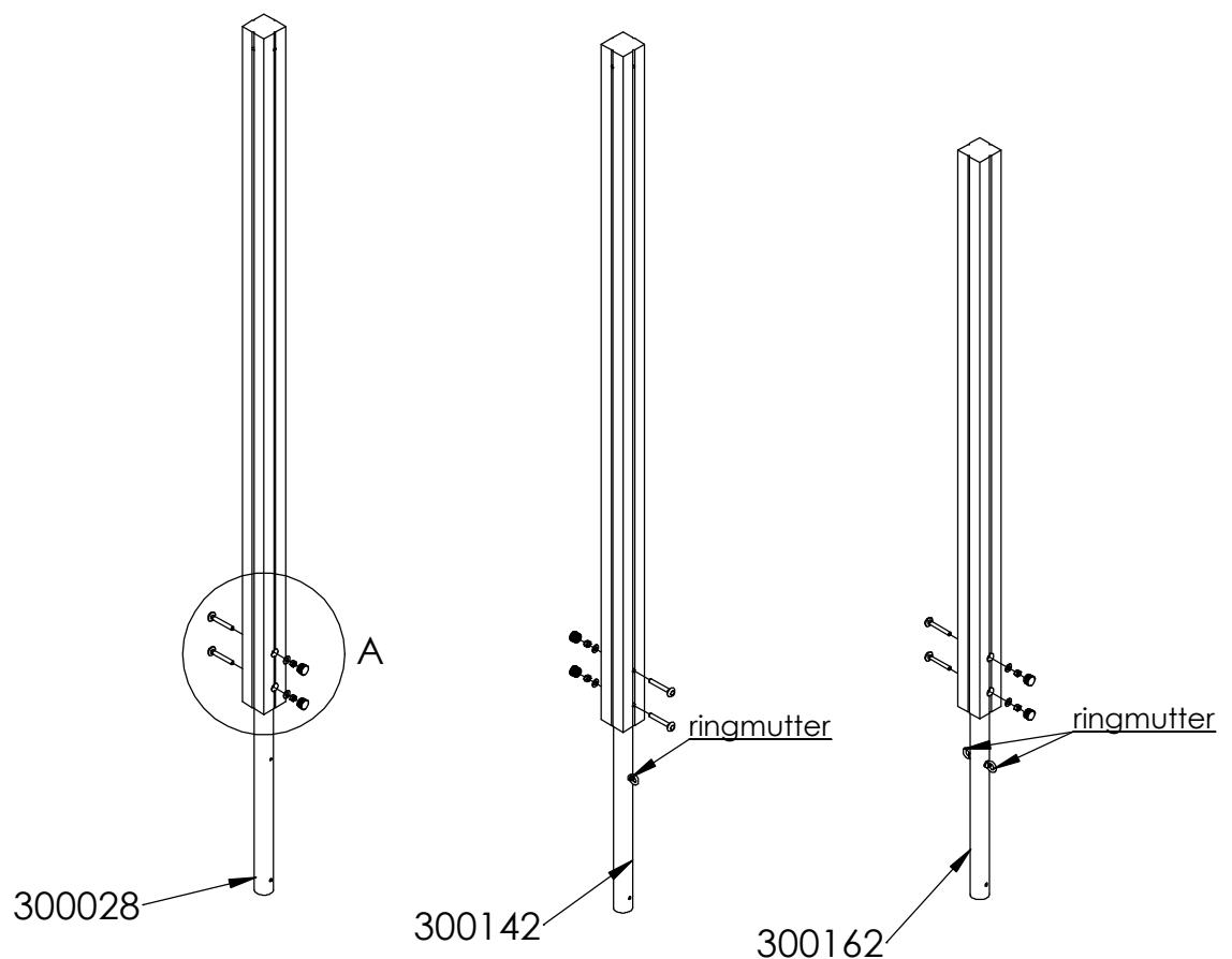
Jordankare art nr 300142 1 st stolpe 300039H 1 st stolpe 300038
