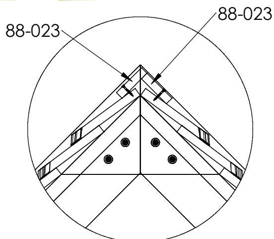
DETAIL AI SCALE 1 : 10
