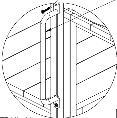
DETAIL AI SCALE 1 : 10
