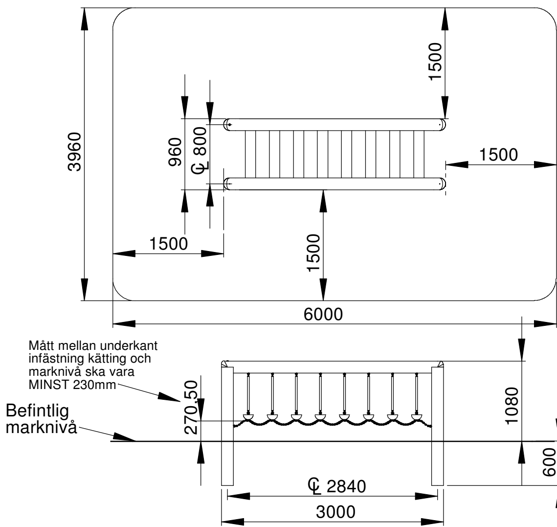
Støpning / Gjutningsdetalj Rundstock Ø180mm
