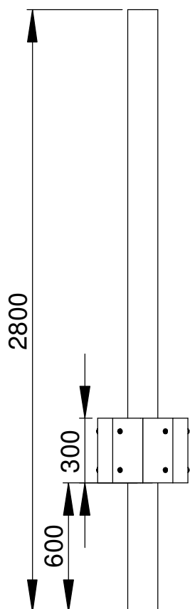
9621-1 Rundstock Förmonterad
