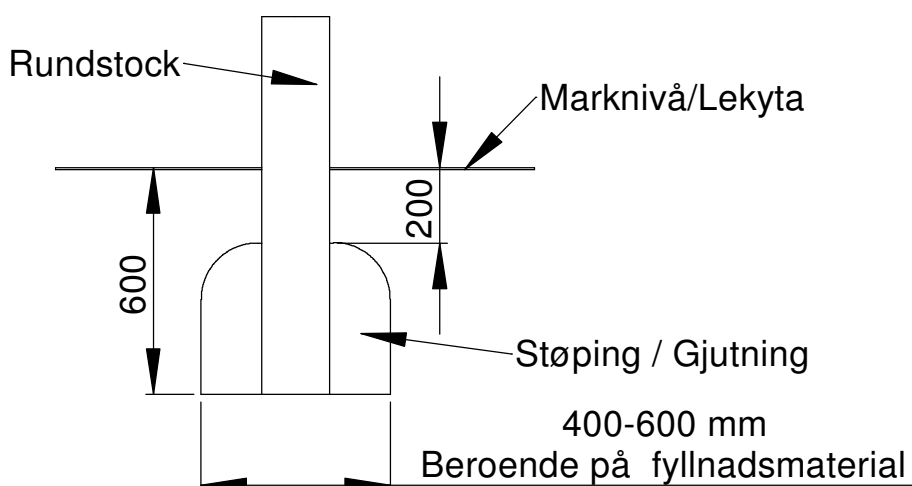
Støping / Gjutningsdetalj Rundstock
