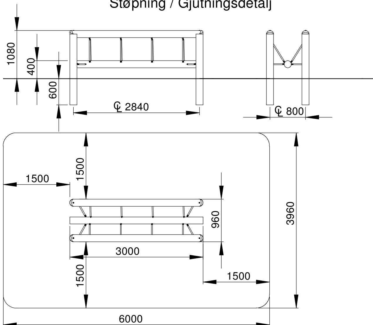
Støpning / Gjutningsdetalj Rundstock Ø180mm
