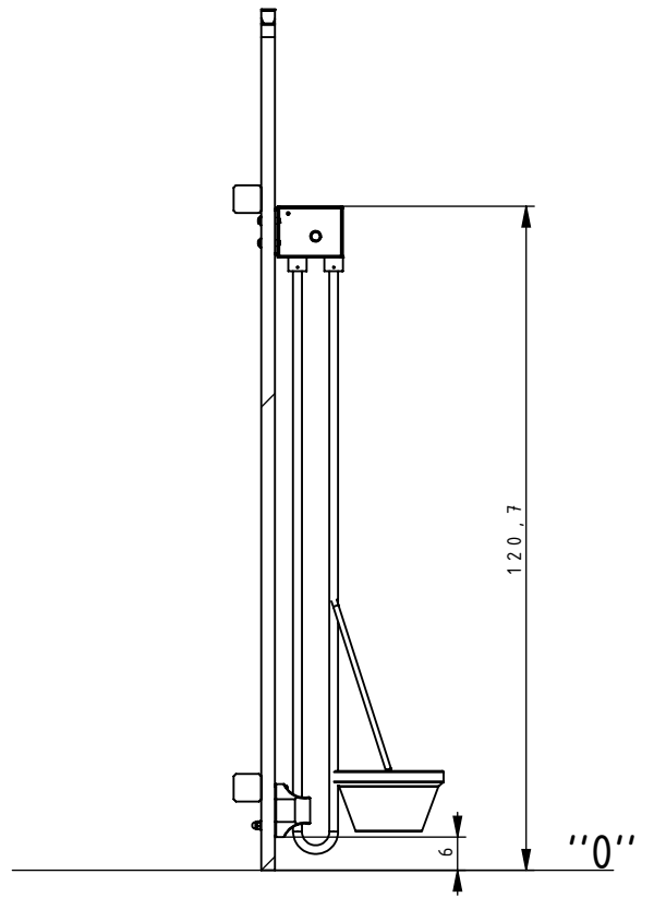
G-G (1 : 15)
