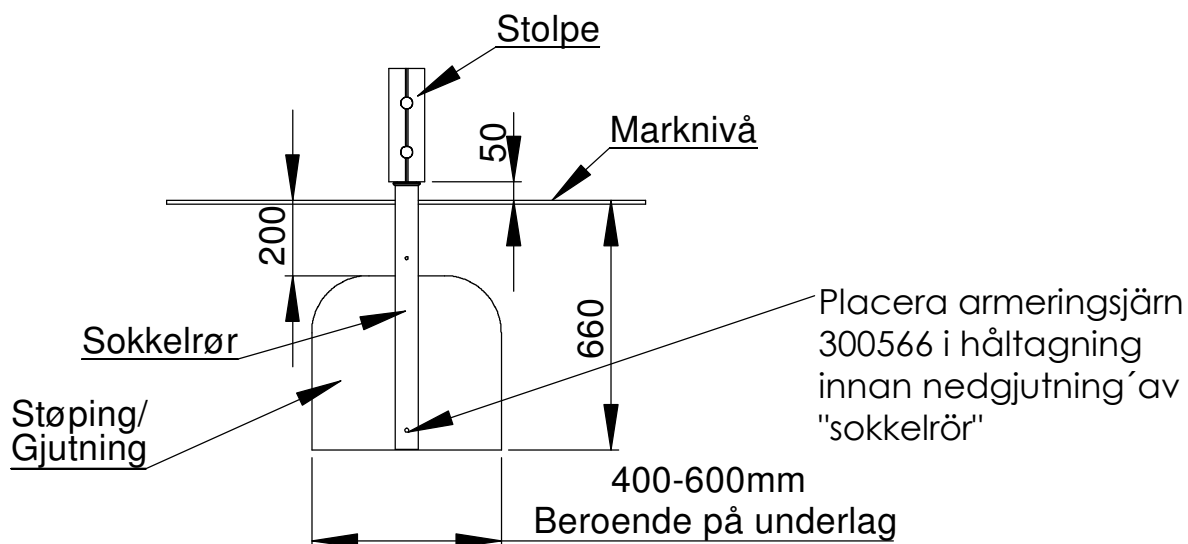
Støping / Gjutningsdetalj
