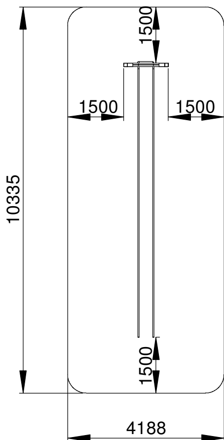
Støping / Gjutningsdetalj
